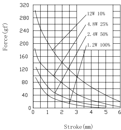
STROKE Vs FORCE 行程/吸引力
