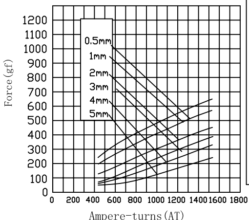
STROKE Vs FORCE 行程/吸引力
